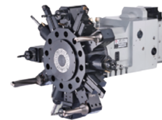
• BMT Live turret
